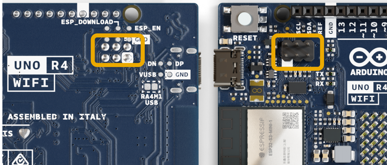
ESP header.
