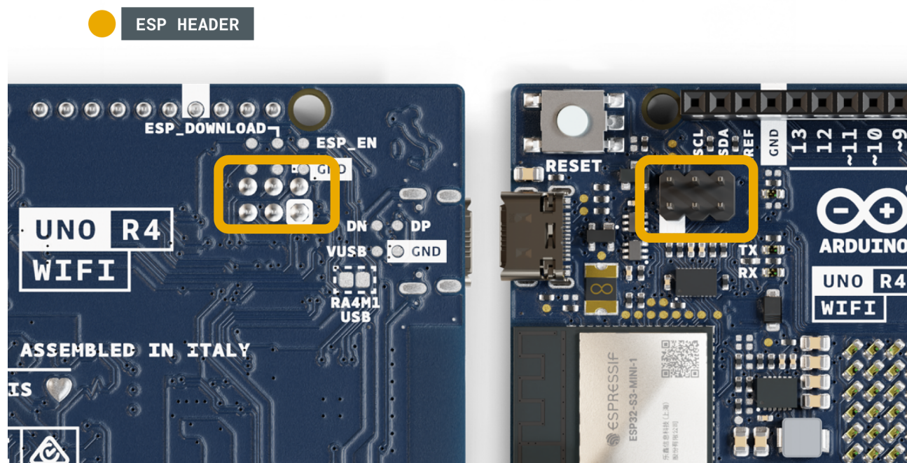
ESP引脚
